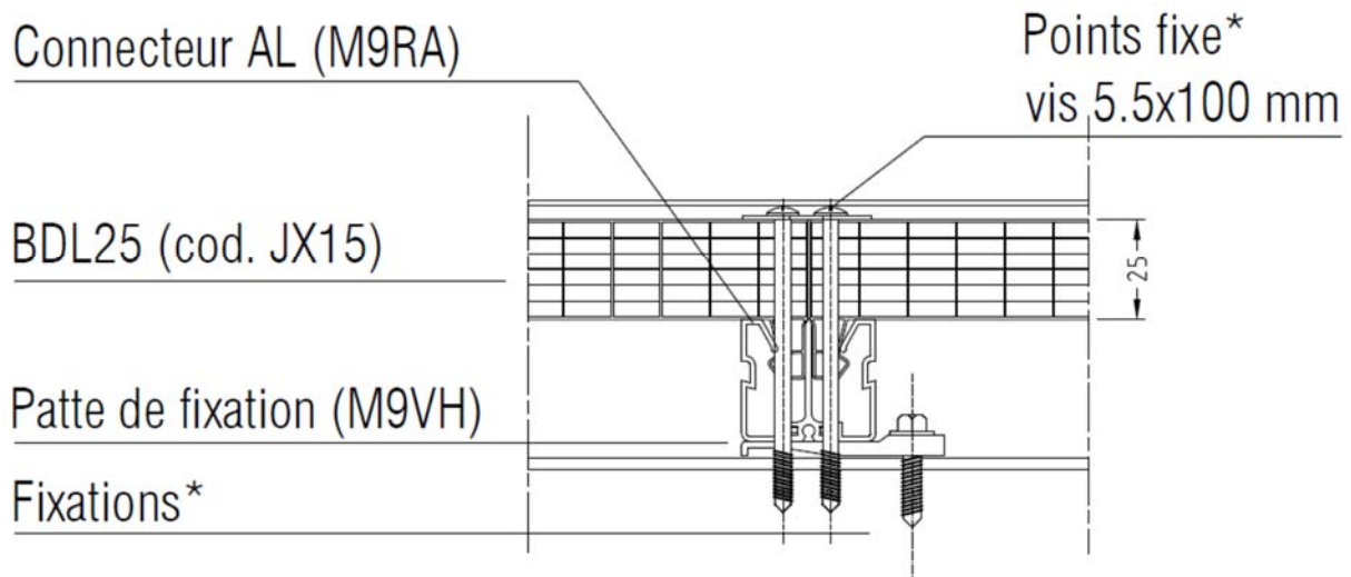
Figure 38 – Position en section point fixe - Pose avec point fixe haut
