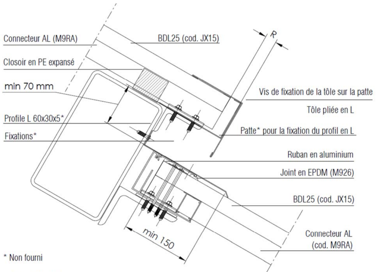
Figure 44 – Ressaut - Pose avec point fixe haut
