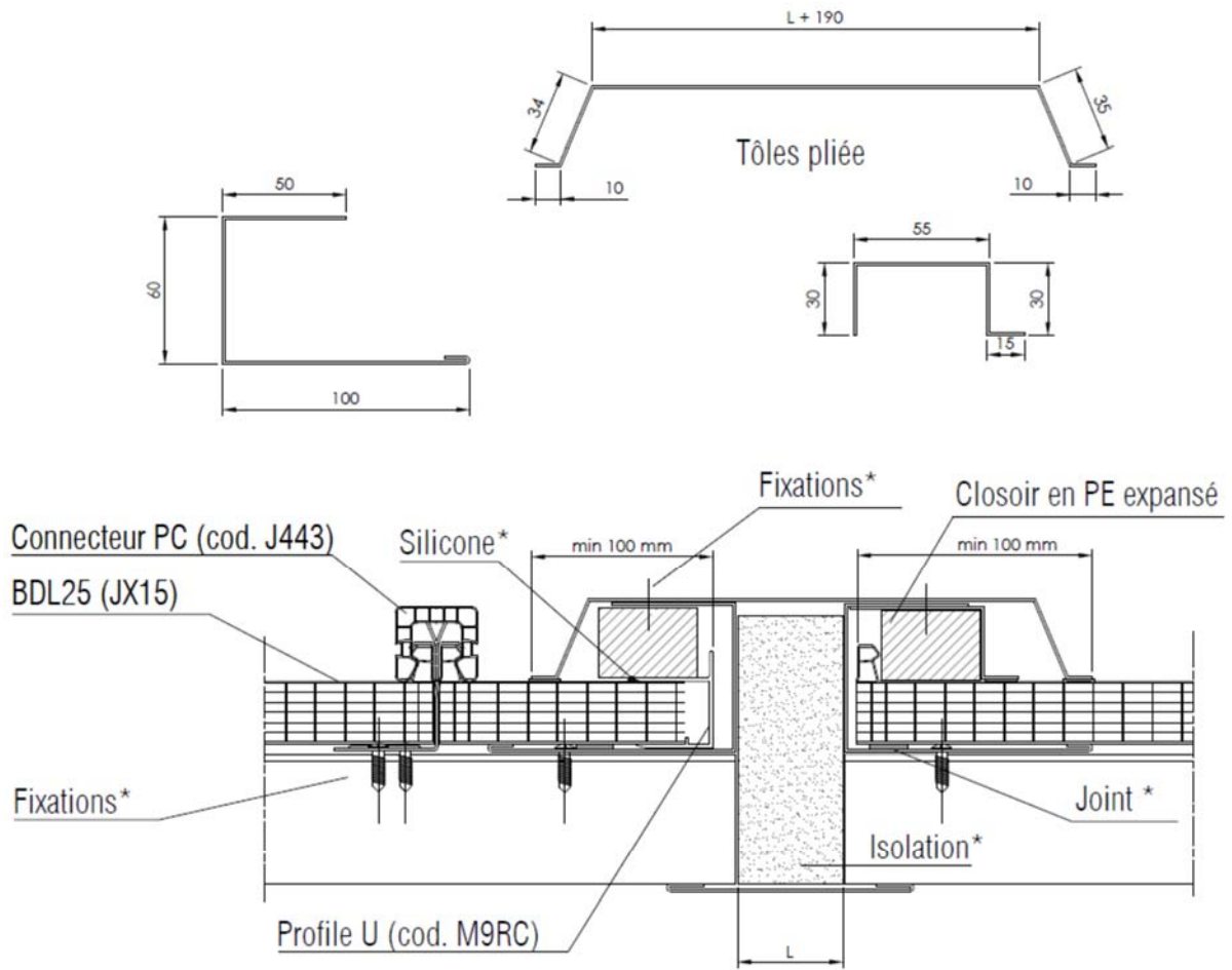
Figure 19 – Joint de dilatation (dans le cas à gauche de bâtiments ouverts uniquement)
