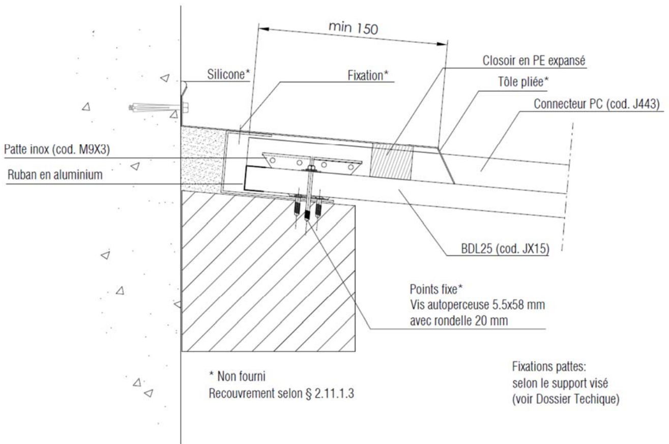
Détail C
