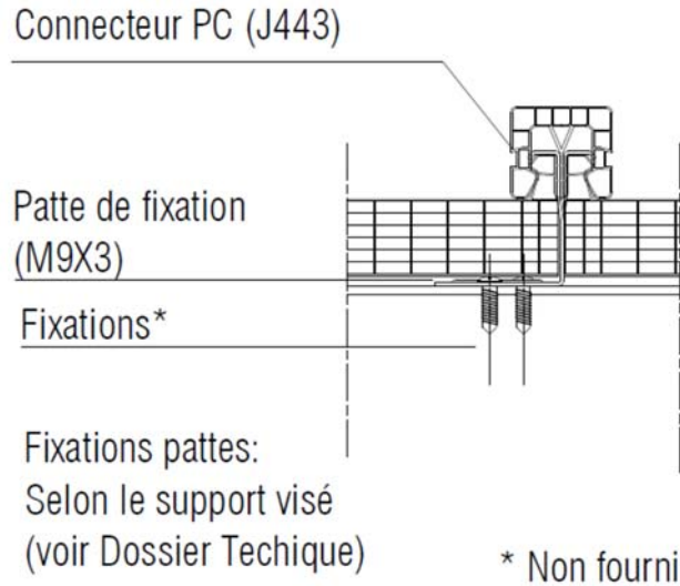
Figure 15 – Égout - Pose avec point fixe bas
