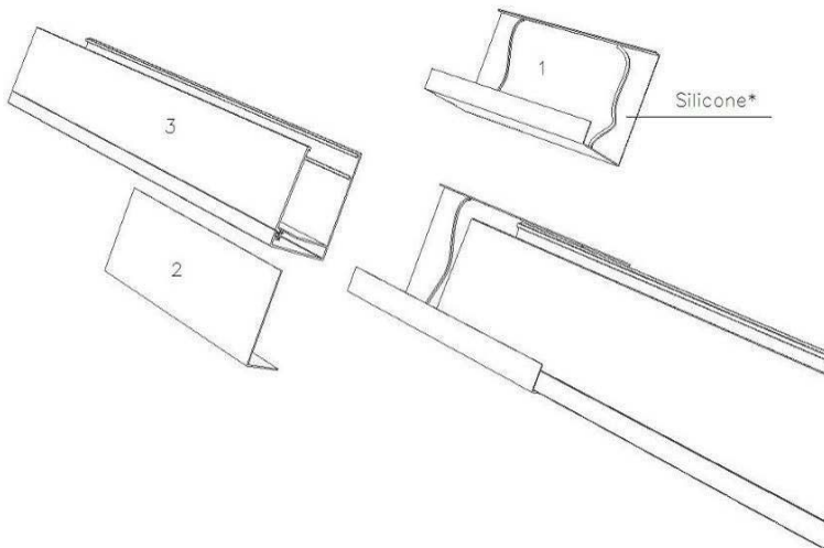
Figure 11 – Aboutage des profils périphériques
