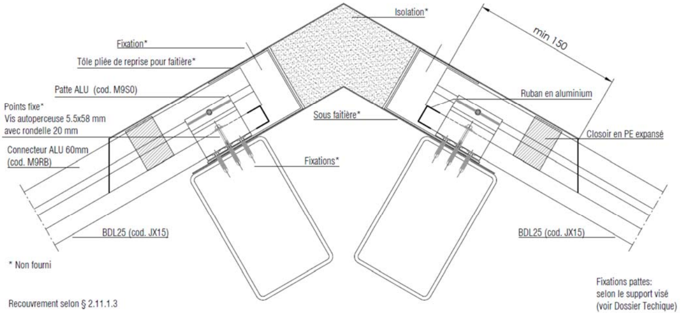
Figure 27j – Faitage double avec point fixe haut et connecteur M9RB
