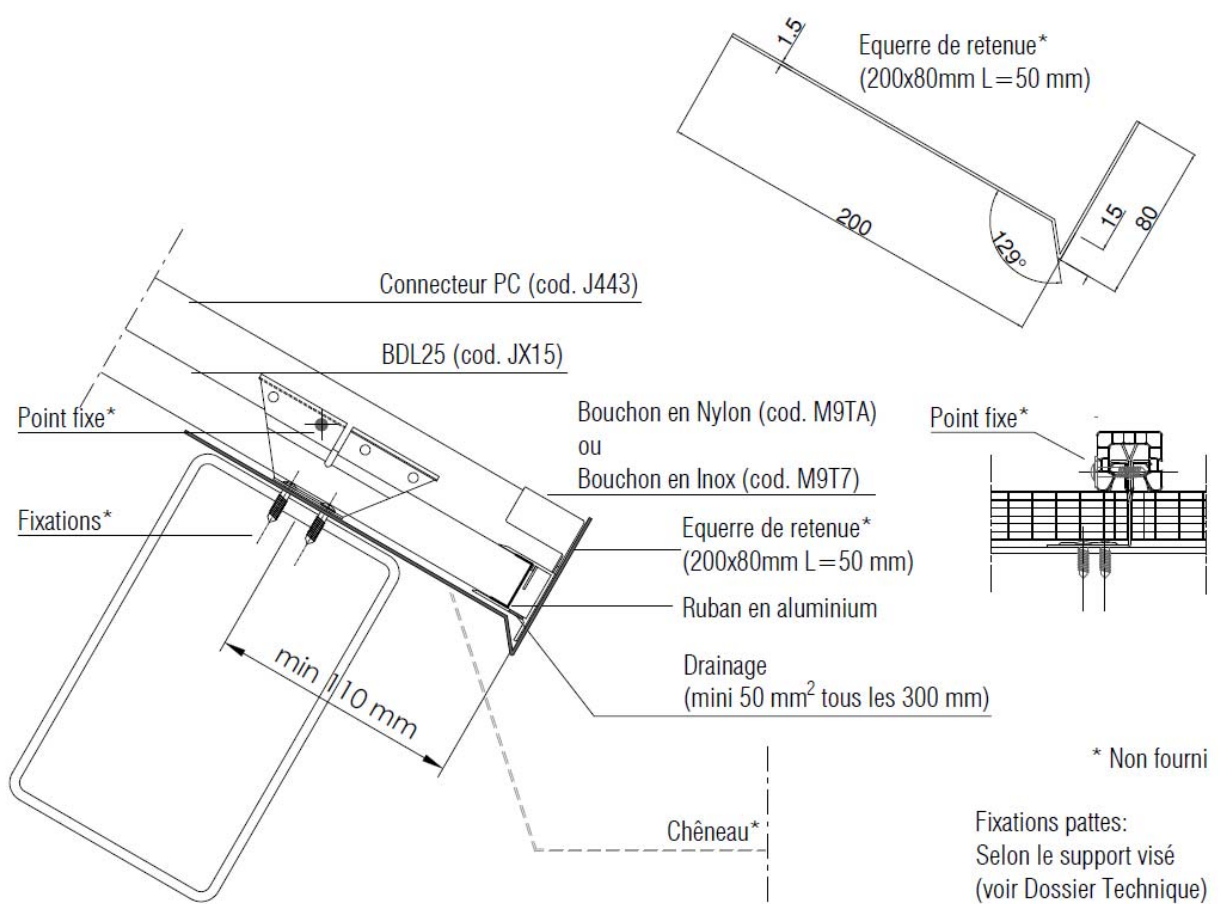
Figure 15 – Égout - Pose avec point fixe bas
