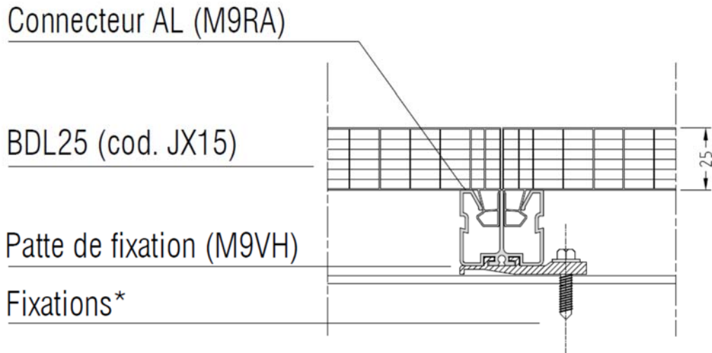
Figure 40– Support intermédiaire - Pose avec point fixe haut
