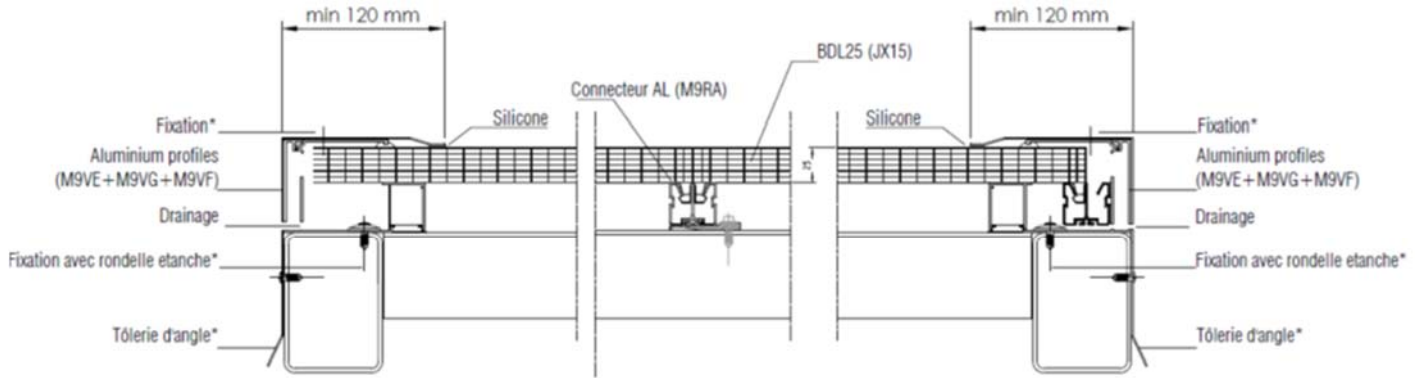
Figure 43 – Raccordement latéral - Pose avec point fixe haut
