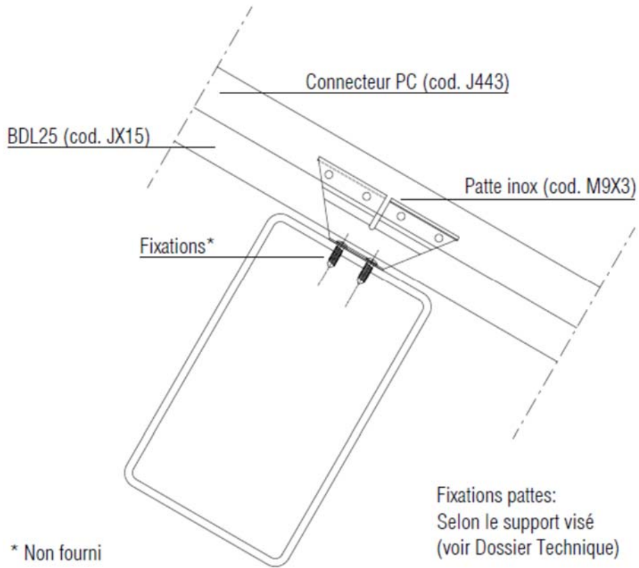
Détail B
