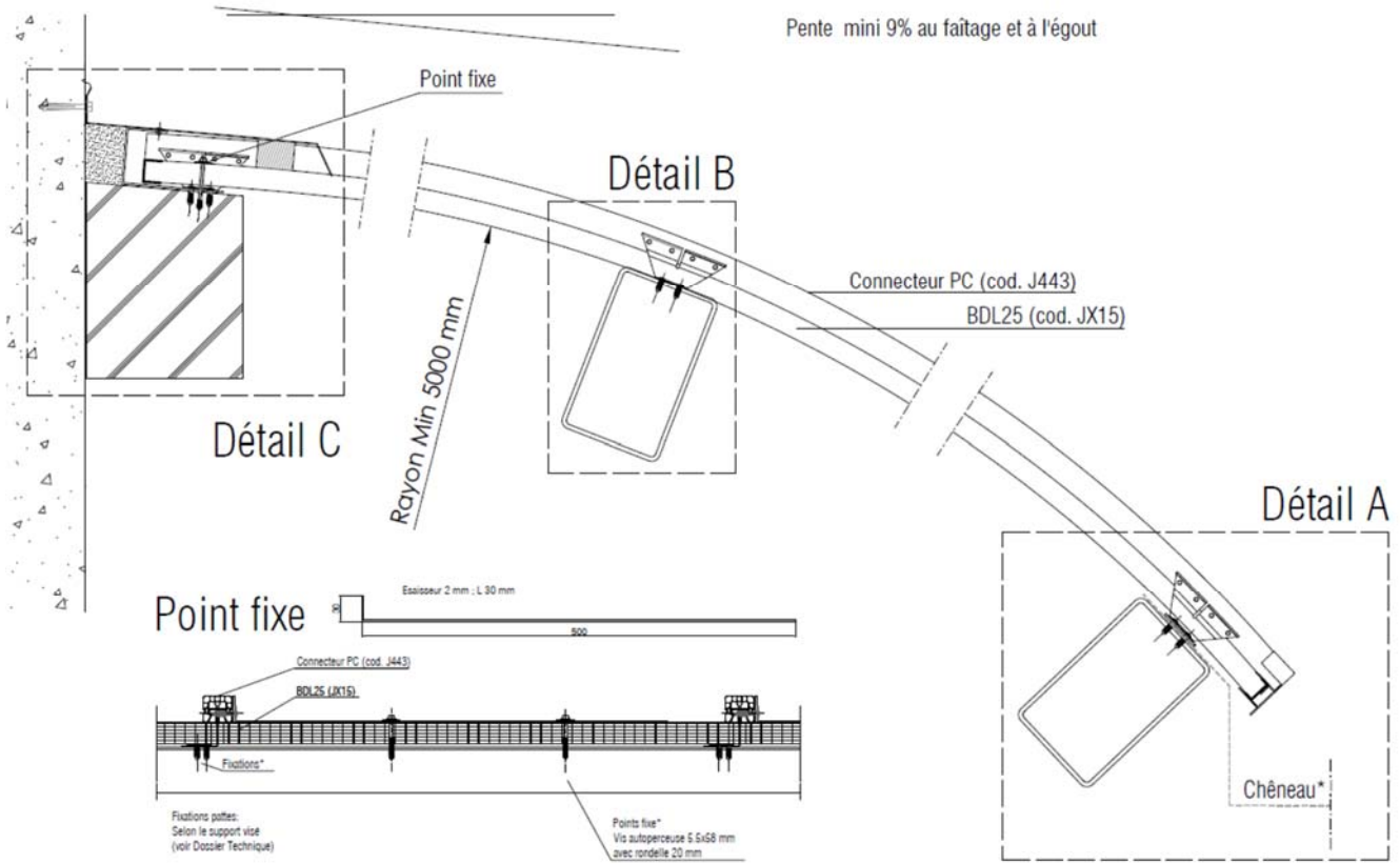
Figure 46 – Pose cintrée en faitage simple ou ½ voûte convexe
